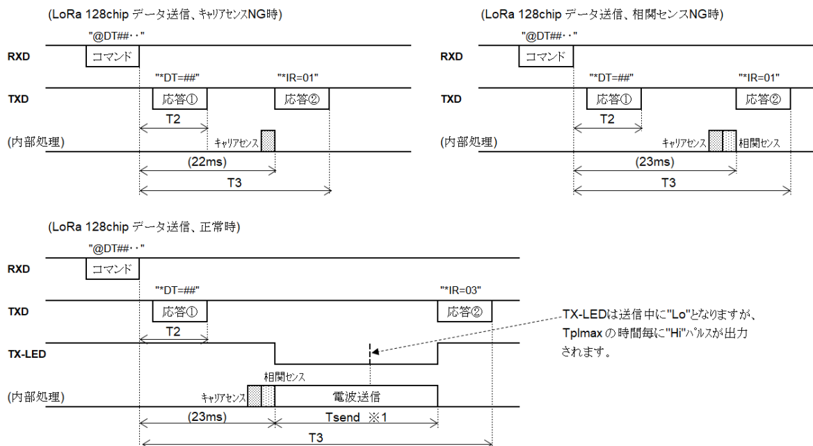
UART 通信速度:19200bps の場合
