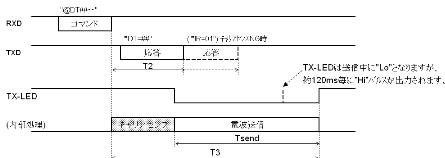
UART 通信速度:19200bps の場合
