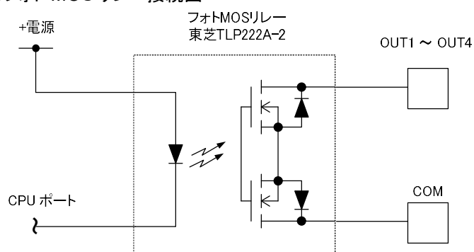
※内部フォト MOS リレー接続図
