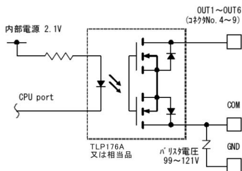
※OUT1～OUT6 出力回路
