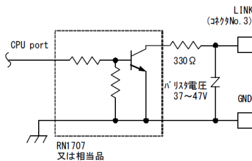
※LINK 出力回路
