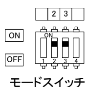
◆出力ボードモードスイッチ設定
