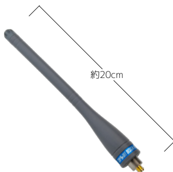
防水アンテナ ANT-400 SMA_MF-20 利得: 2.14dBi以下 全長: 約20cm
